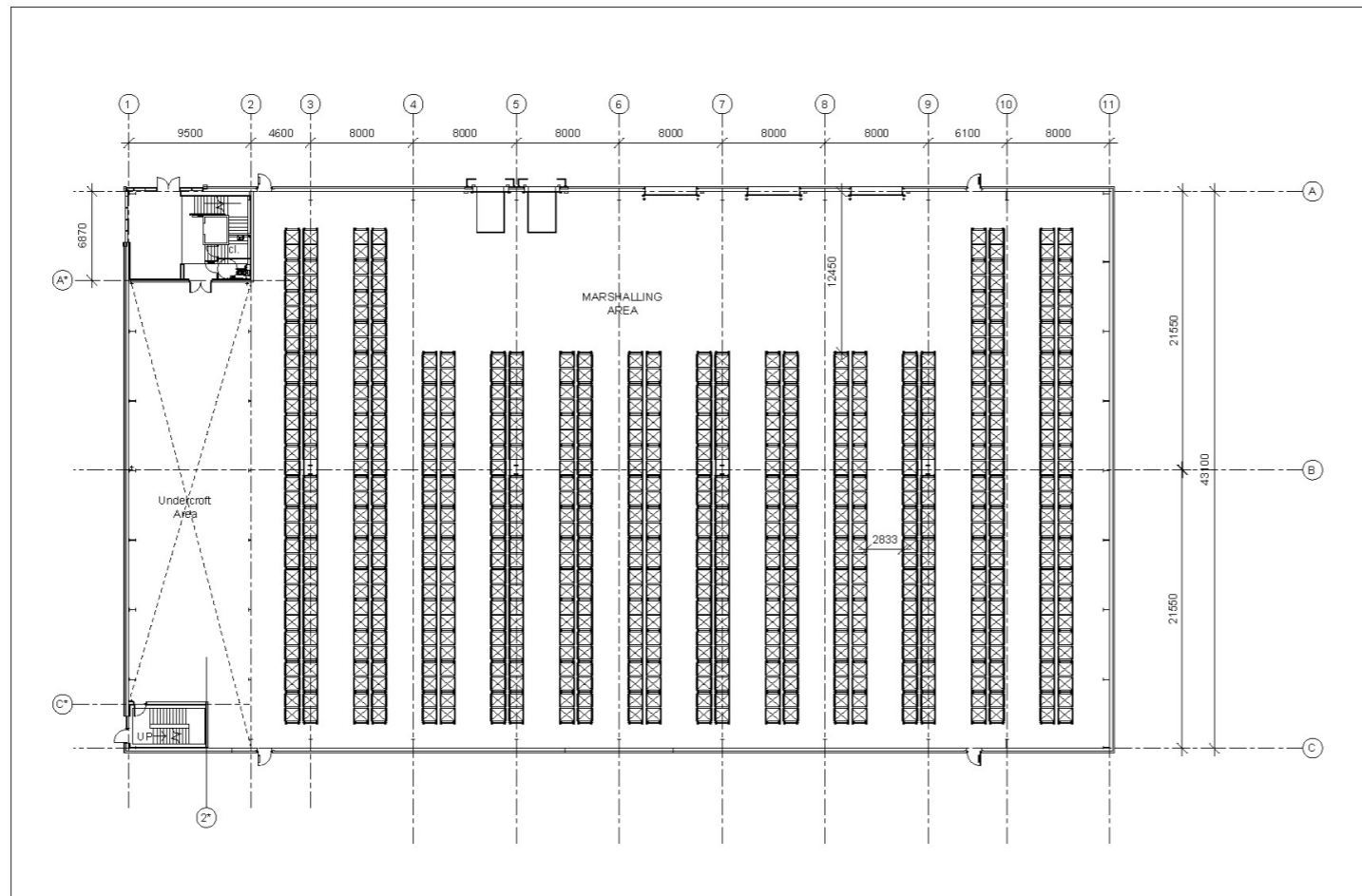
1 Warehouse Plan 1 : 250
