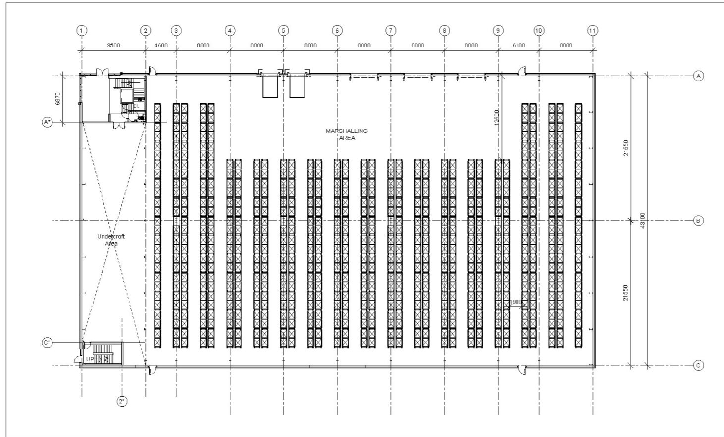
1 Warehouse Plan 1 : 250
